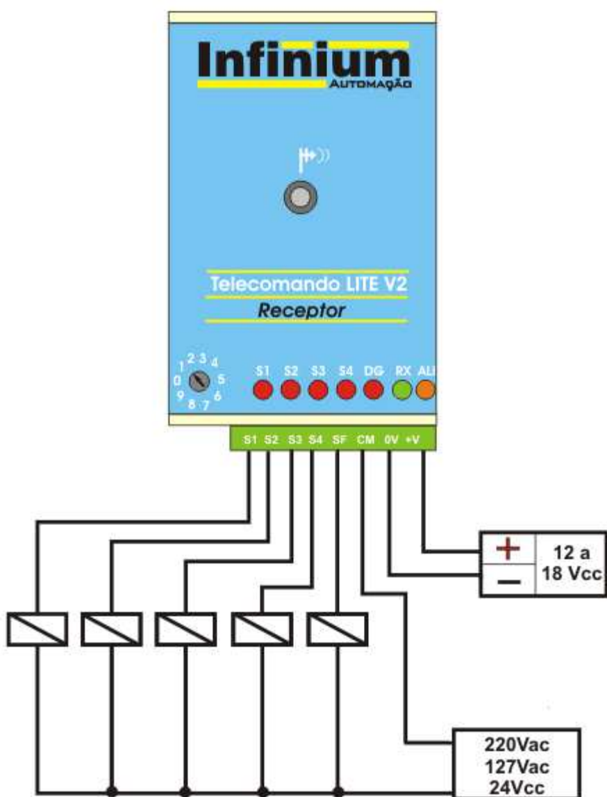
Diagrama de interligação Receptor
