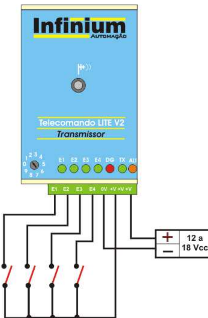
Diagrama de interligação Transmissor
